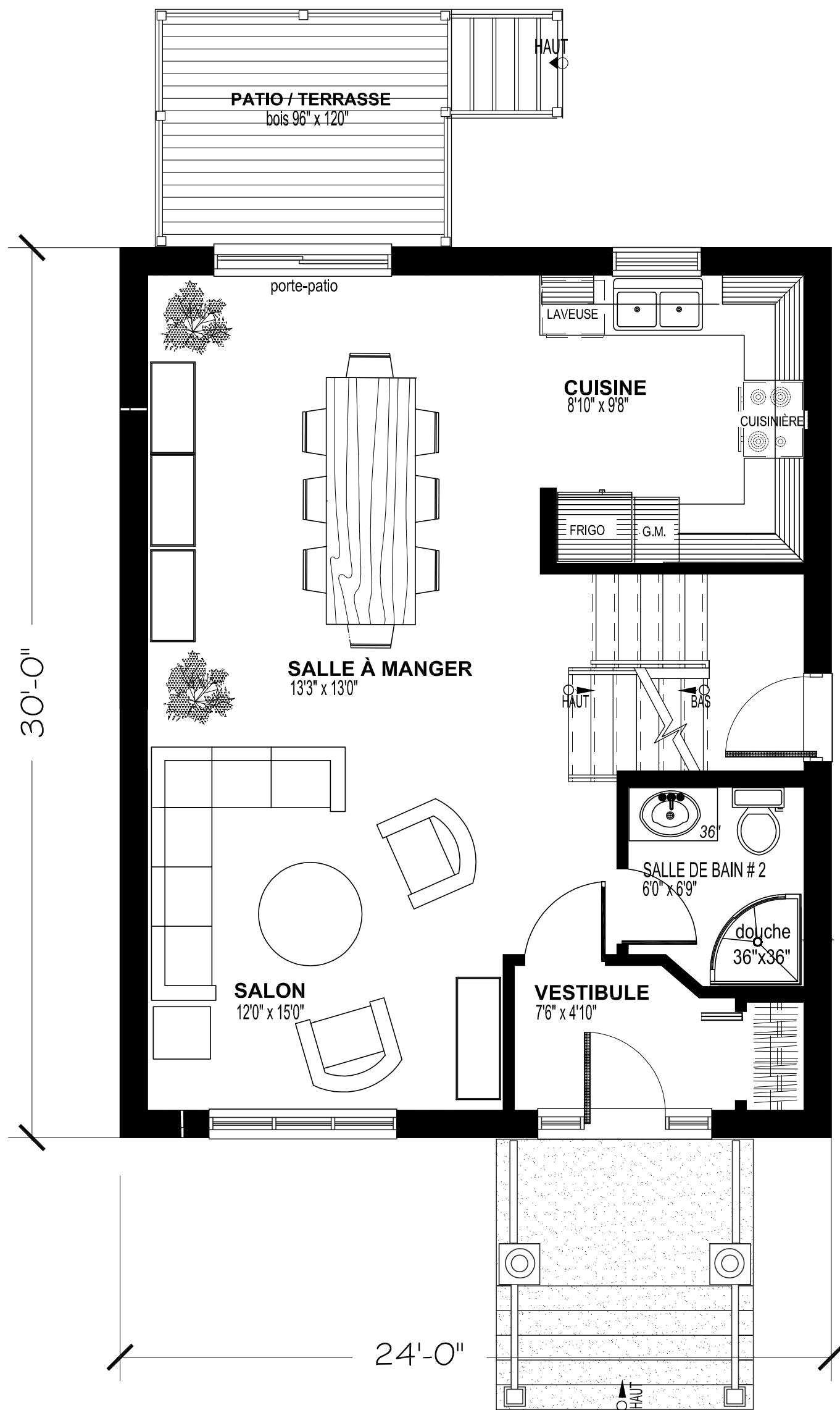
NIVEAU REZ-DE-CHAUSSÉE MODÈLE "ADAGIO "
