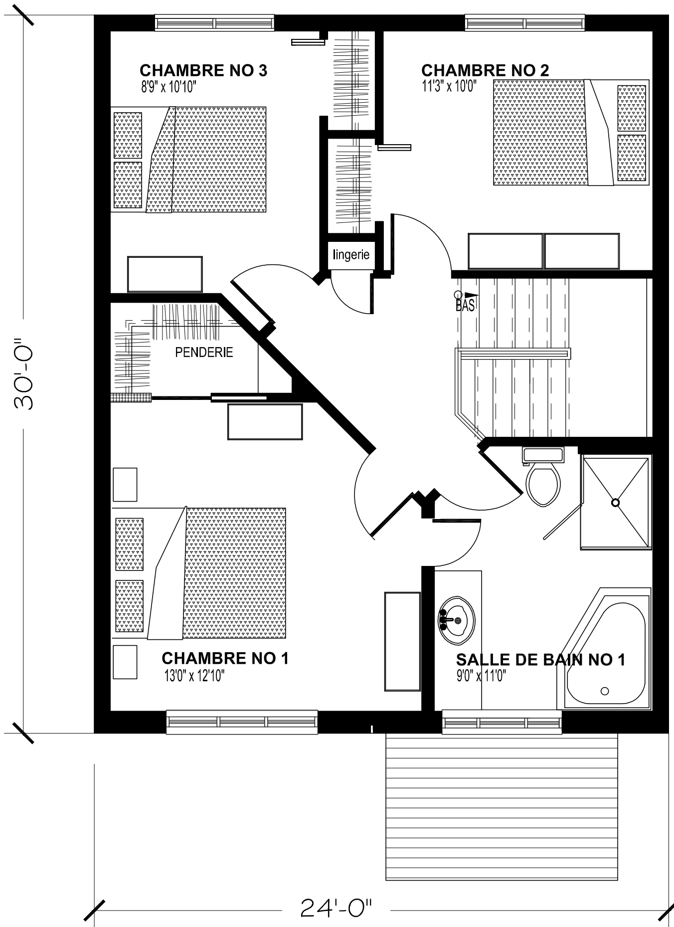
NIVEAU : PREMIER ÉTAGE MODÈLE "ADAGIO "
